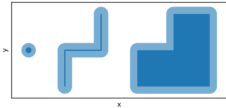
s.buffer(0.2)
