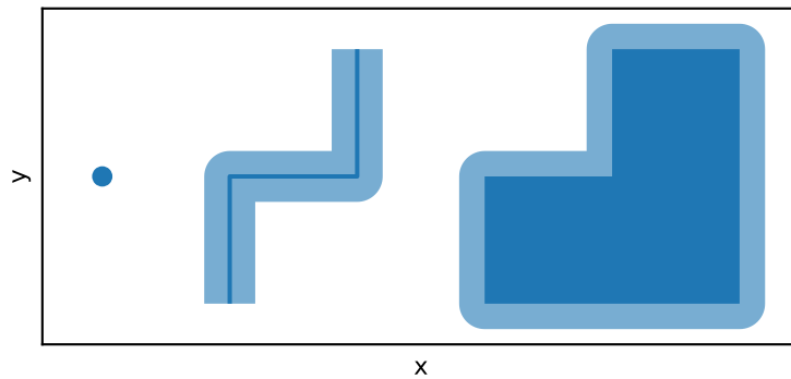
s.buffer(0.2, cap_style="flat")
