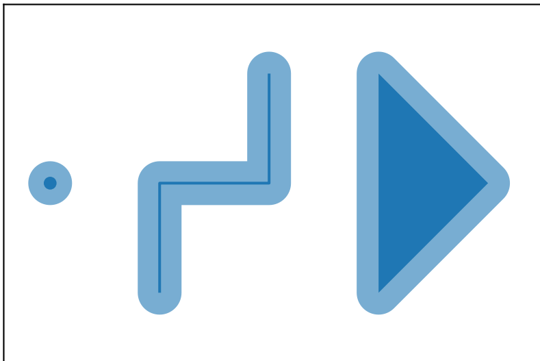
s.buffer(0.2)
