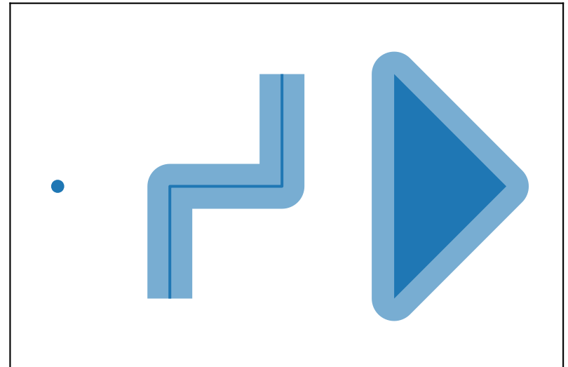
s.buffer(0.2, cap_style="flat")
